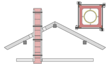
Stand sicherheitskonstruktion aus verzinkten Stahlwinkeln und Umspannungsbändern
